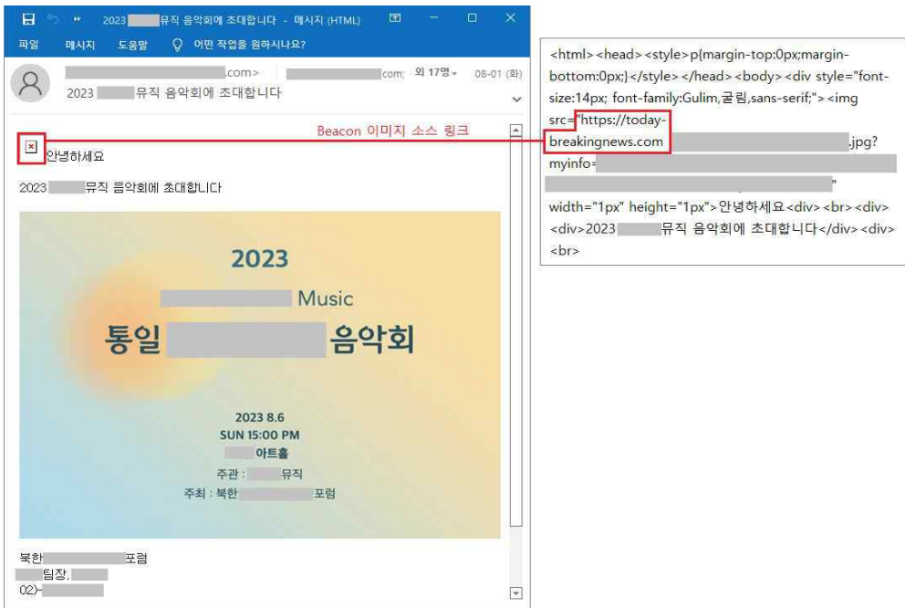
[그림 16] 통일 관련 미약화로 사칭해 현충 중인 메일의 비콘 코드 화면
